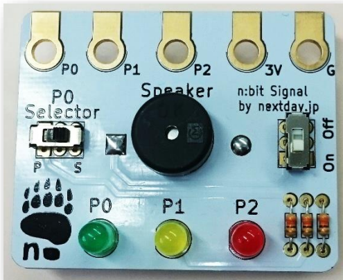
LED信号/SP(スピーカー)基板
